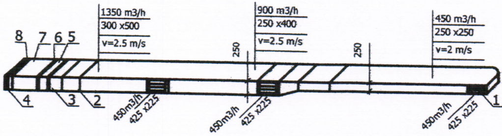
Схема на приточна вентилационна система П-2
